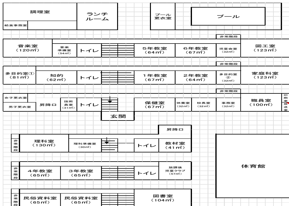
校舎配置図
